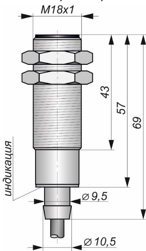
Габаритный чертеж
